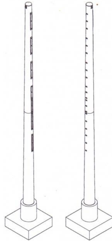
POSTE DE HORMIGÓN DE 28m PARA LÍNEAS DE 115 Y 138 Kv CON DOS CIRCUITOS DE MEDIA TENSION
